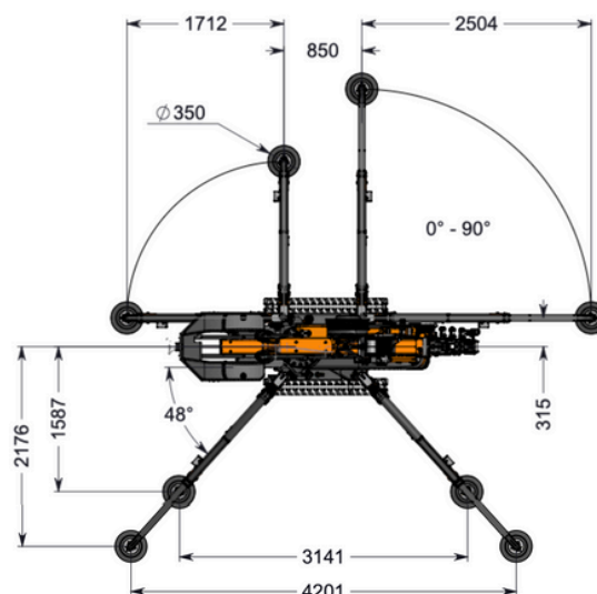
ENCOMBREMENT AU SOL (MM)
